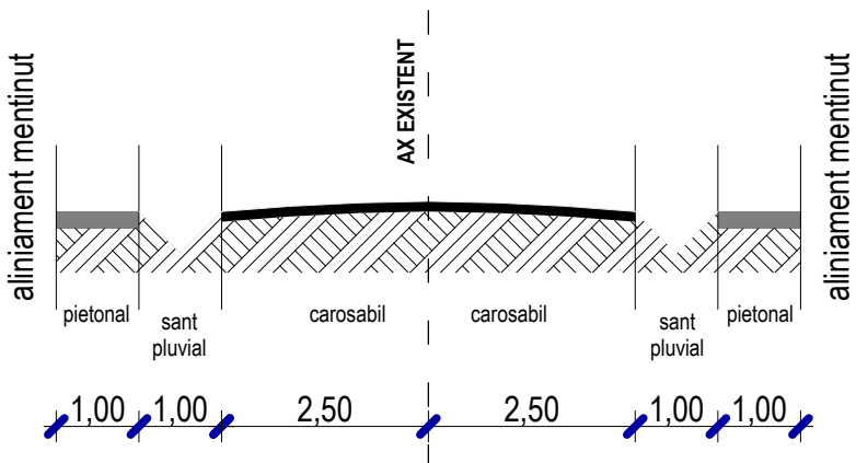
PROFIL MINIM PENTRU STRAZI SECUNDARE SC. 1:100
