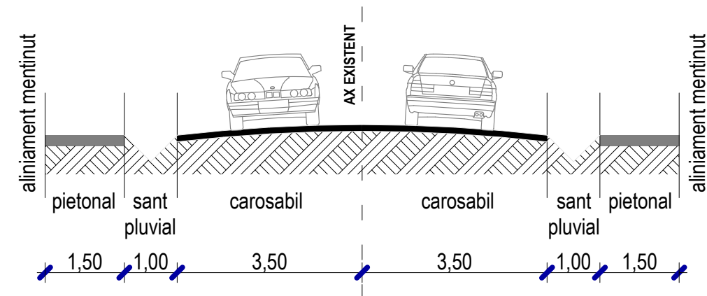
PROFIL MINIM PENTRU STRAZI PRINCIPALE SC. 1:100
